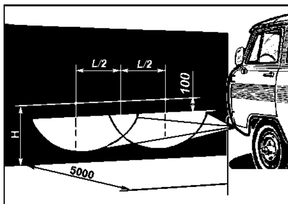
Рис. 9.40. Разметка экрана для регулировки противотуманных фар:
