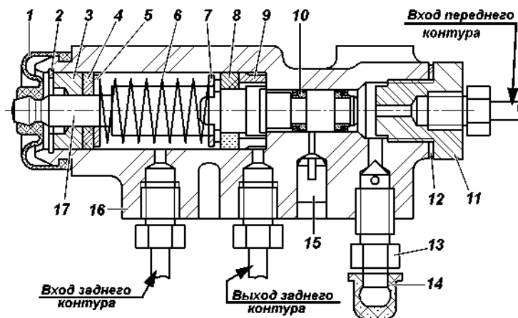
Рис. 9.30. Регулятор давления:
