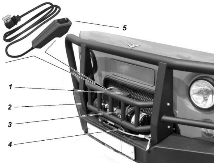
Рис. 10.3. Лебедка:
