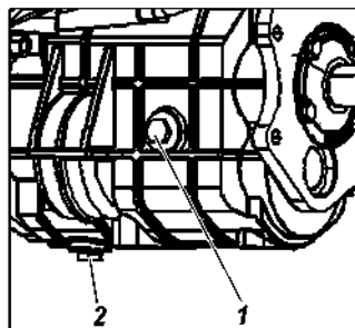
Рис. 9.13. Пробки коробки передач: 1 -пробка заливного отверстия; 2 -пробка сливного отверстия
